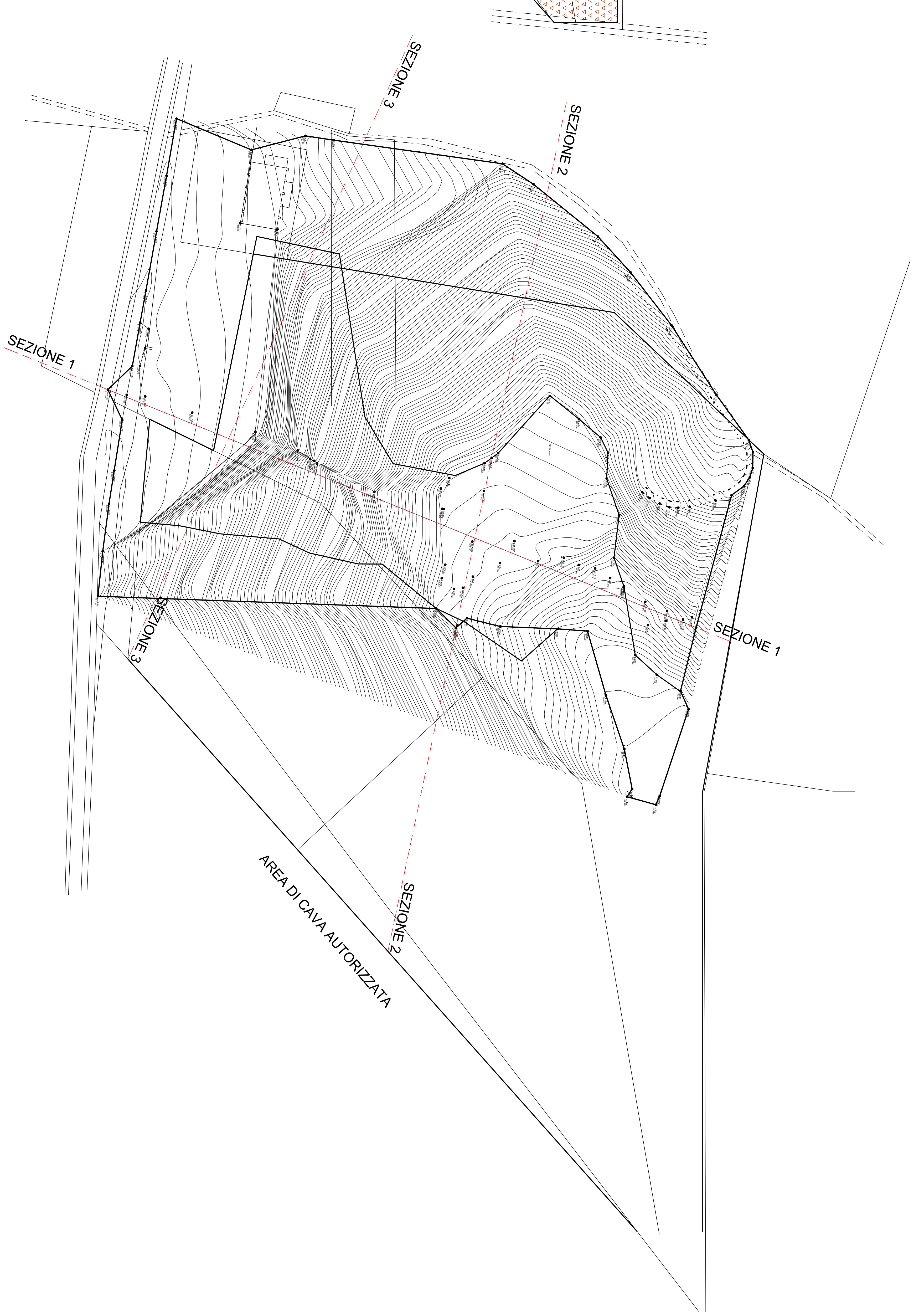
Piano Quotato sc. 1:1000
