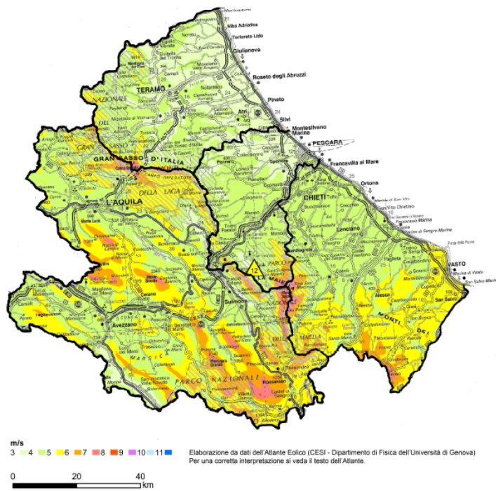
Figura 1: Velocità media annua del vento a 50 metri s.l.m. in Abruzzo (fonte Atlante Eolico dell'Italia- Cesi, Dipartimento di Fisica dell'Università di Genova)
