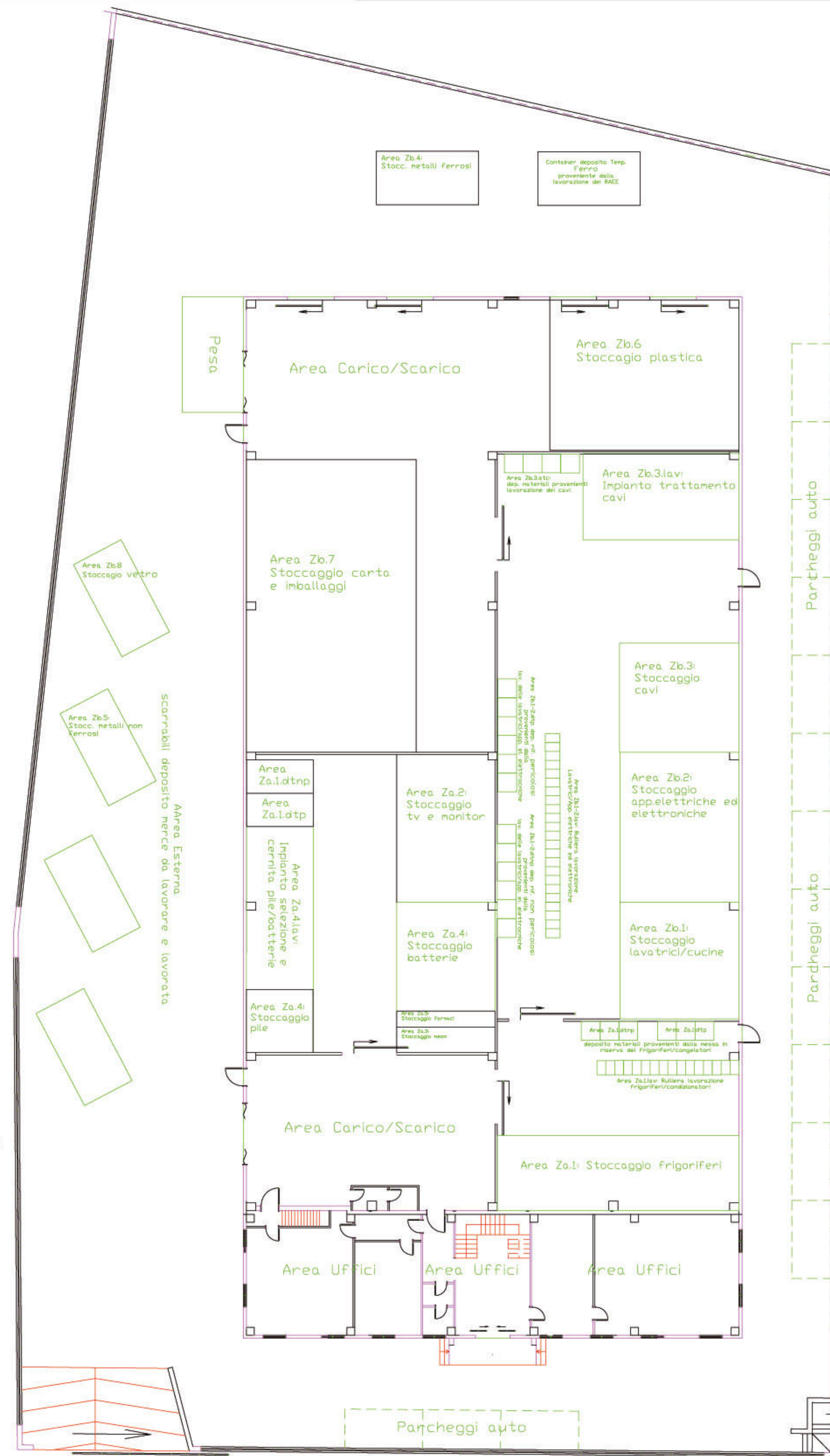
LAYOUT IMPIANTO scala 1:100
