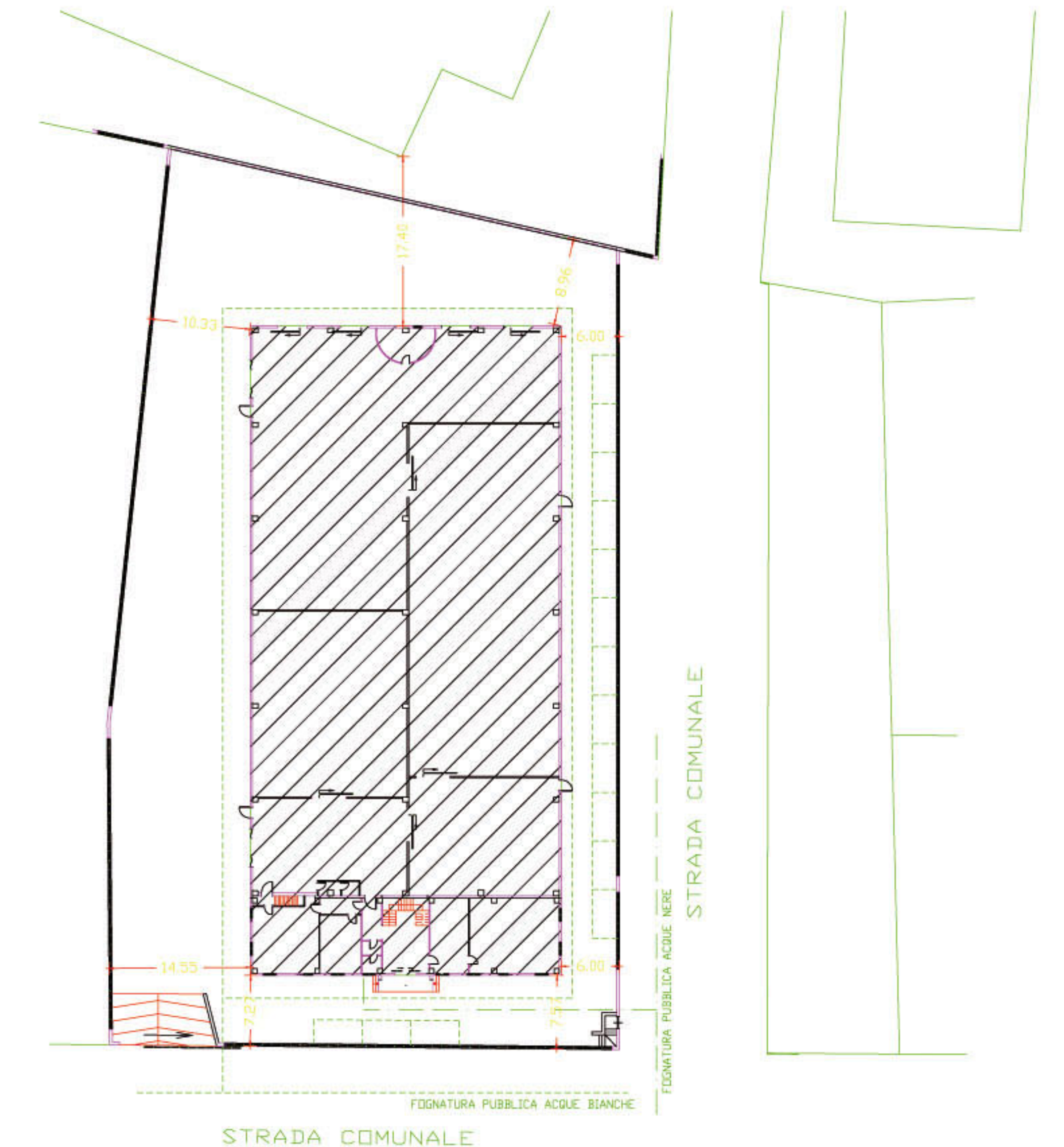
PLANIMETRIA scala 1:500
