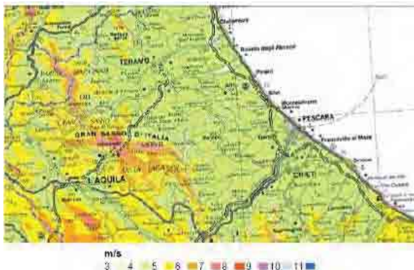
Figura 4 - Mappa della velocità del vento media annua a 70 m s.l.m.
